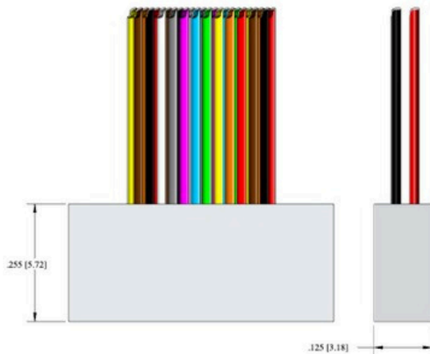
RECEPTACLE (SOCKETS)
