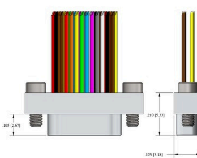
PLUG (PINS)
