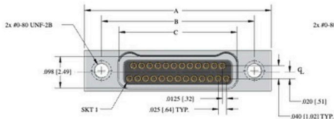
RECEPTACLE (SOCKETS)
