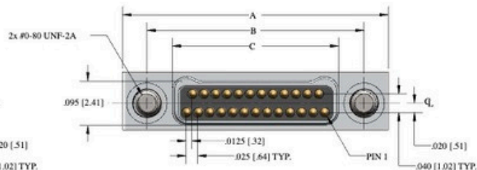
PLUG (PINS)
